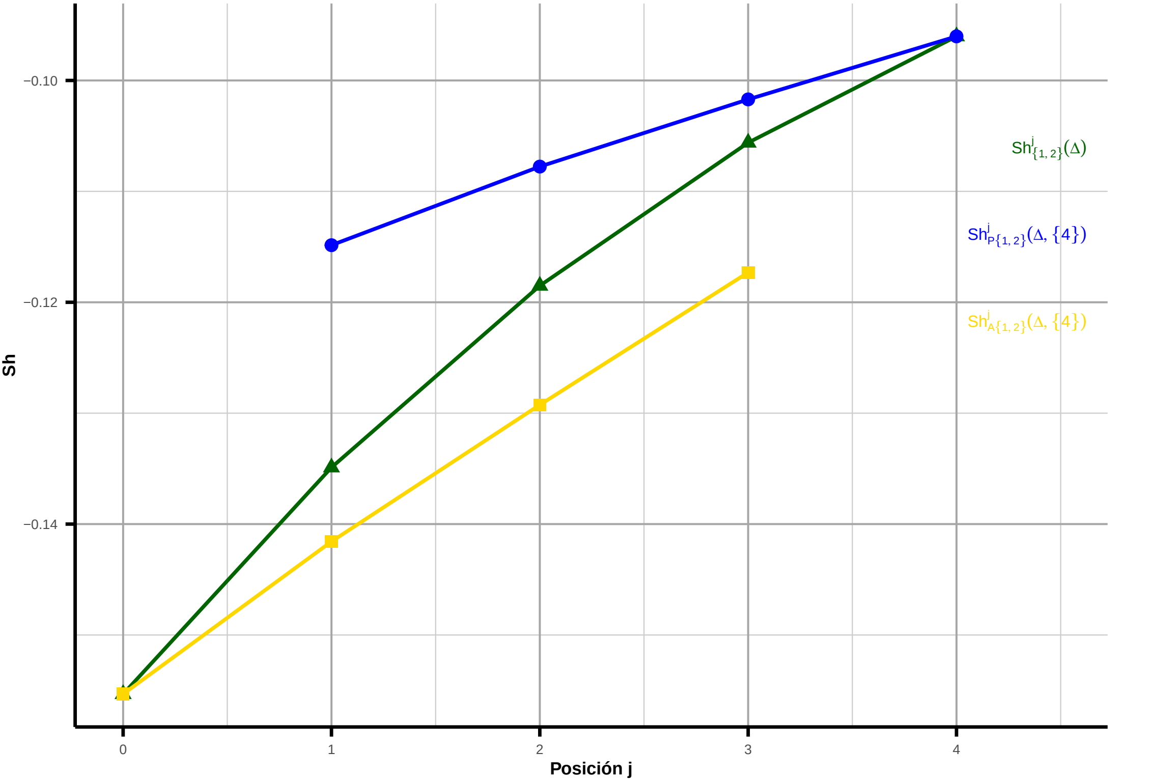
Influencia de Ris [4] sobre Age + Cho [1,2] (instancia fila = 1)
