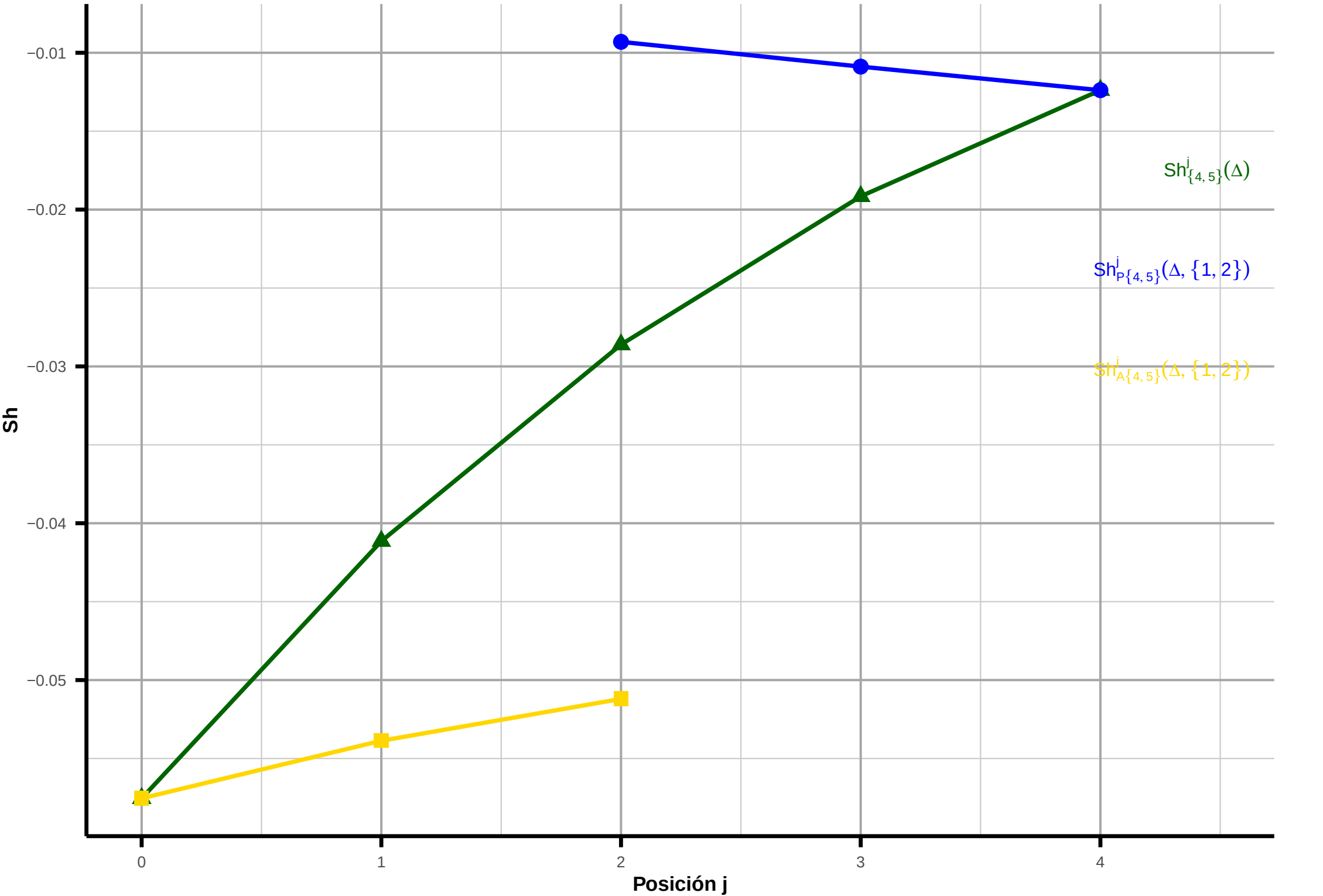
Influencia de Age + Cho [1,2] sobre Ris + Sex [4,5] (instancia fila = 1)
