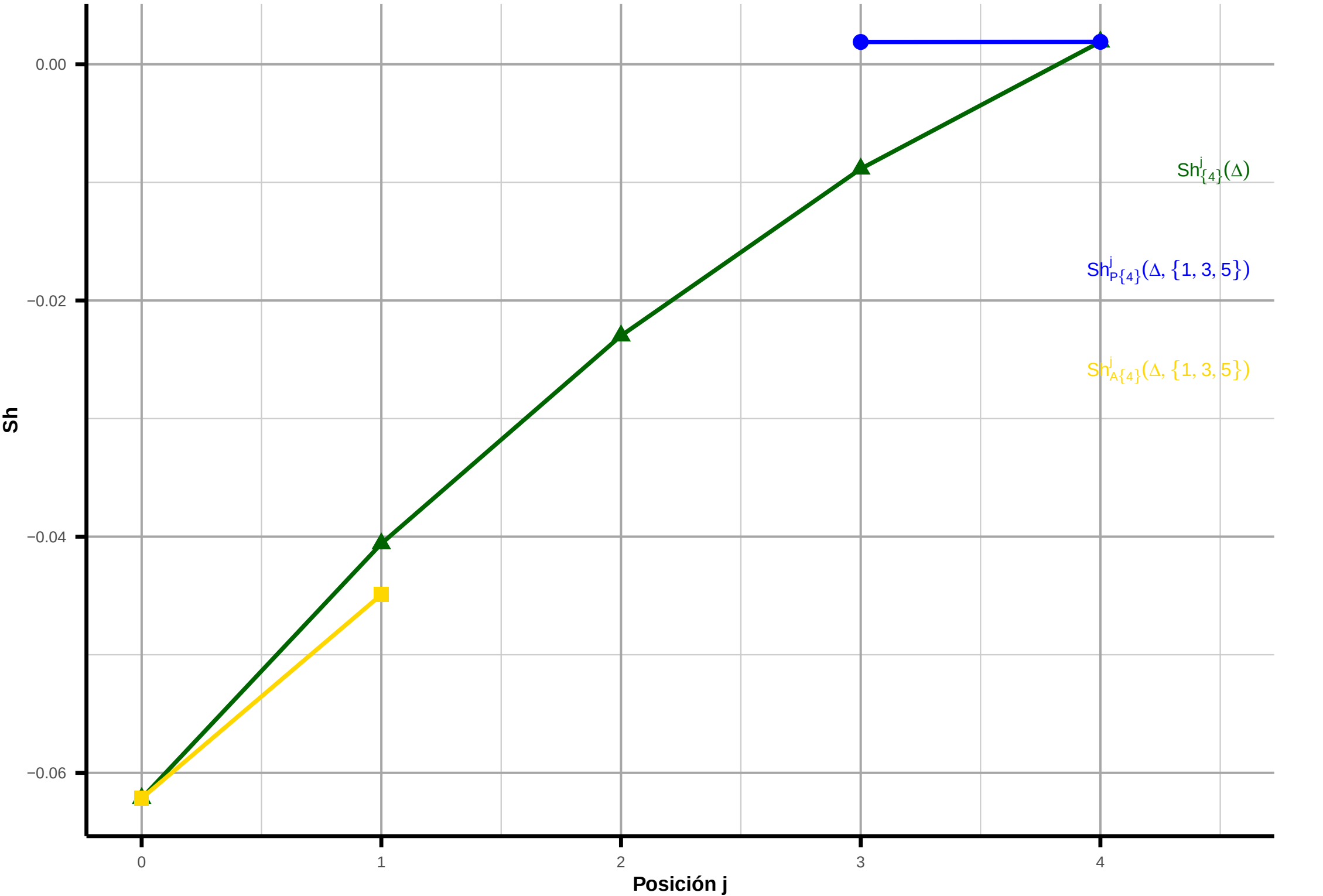
Influencia de Age + Rac + Sex [1,3,5] sobre Ris [4] (instancia fila = 1)
