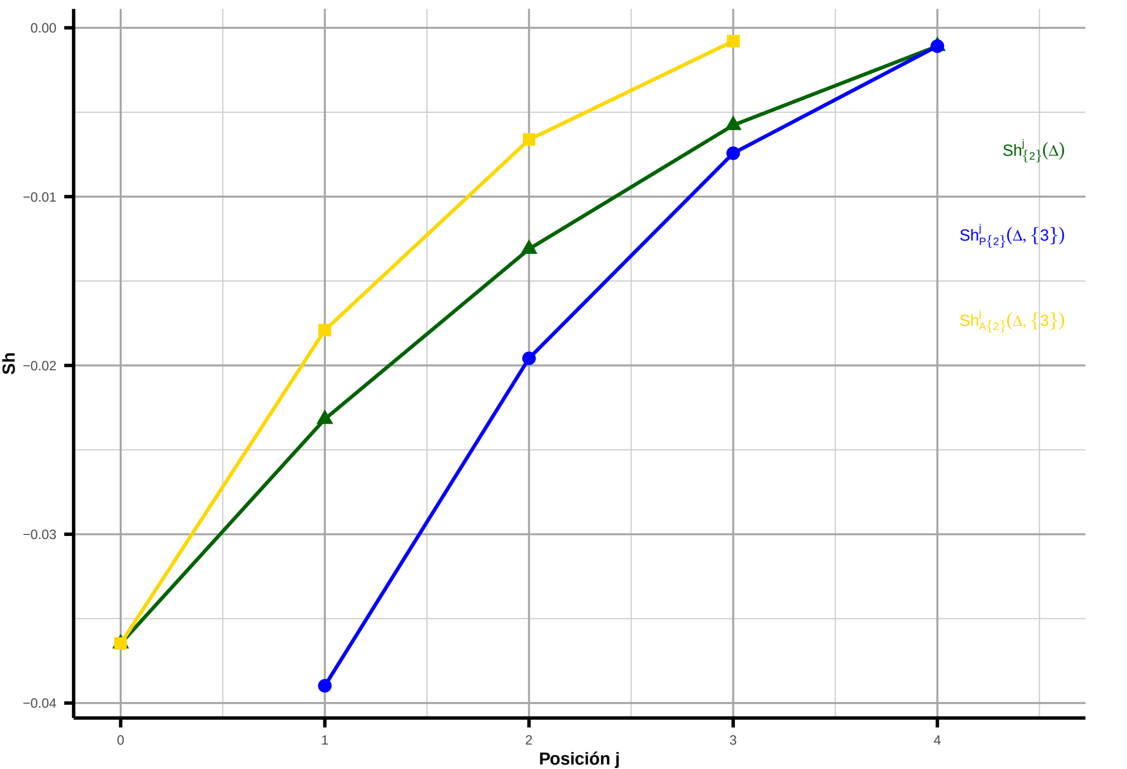
Influencia de Rac [3] sobre Cho [2] (instancia fila = 1)
