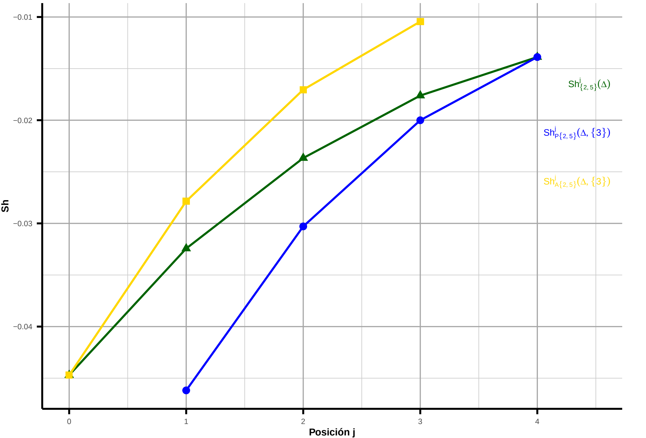
Influencia de Rac [3] sobre Cho + Sex [2,5] (instancia fila = 1)
