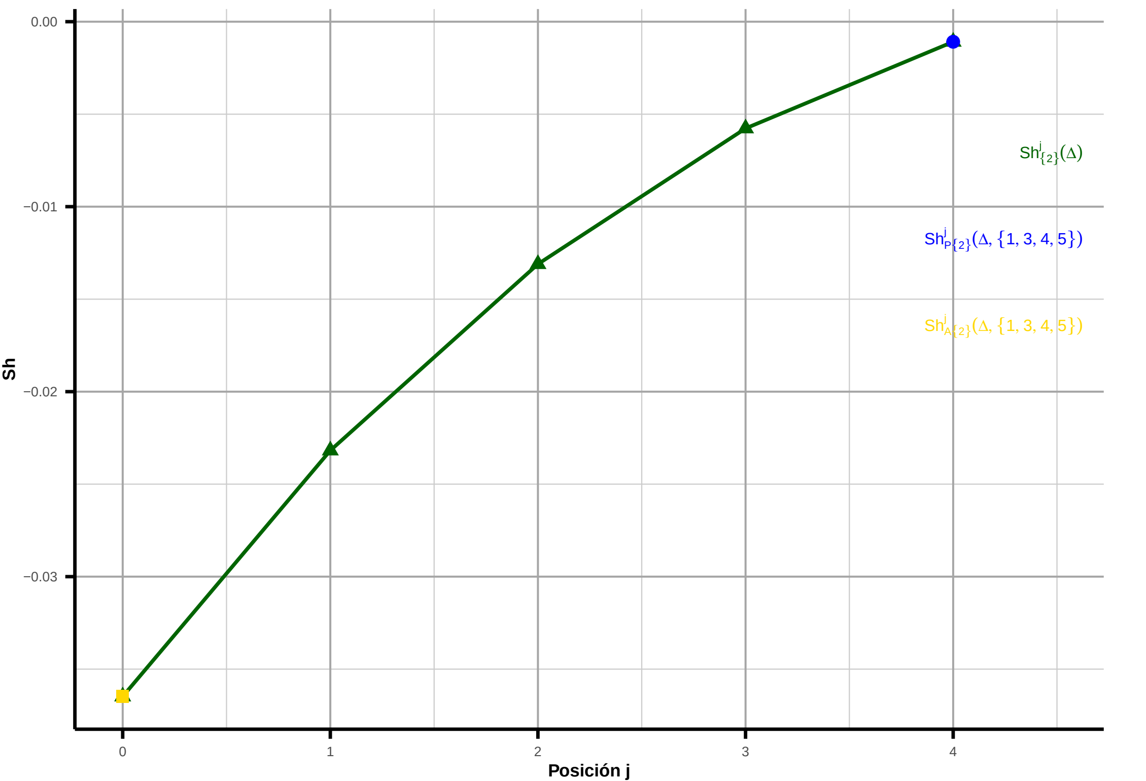
Influencia de Age + Rac + Ris + Sex [1,3,4,5] sobre Cho [2] (instancia fila = 1)
