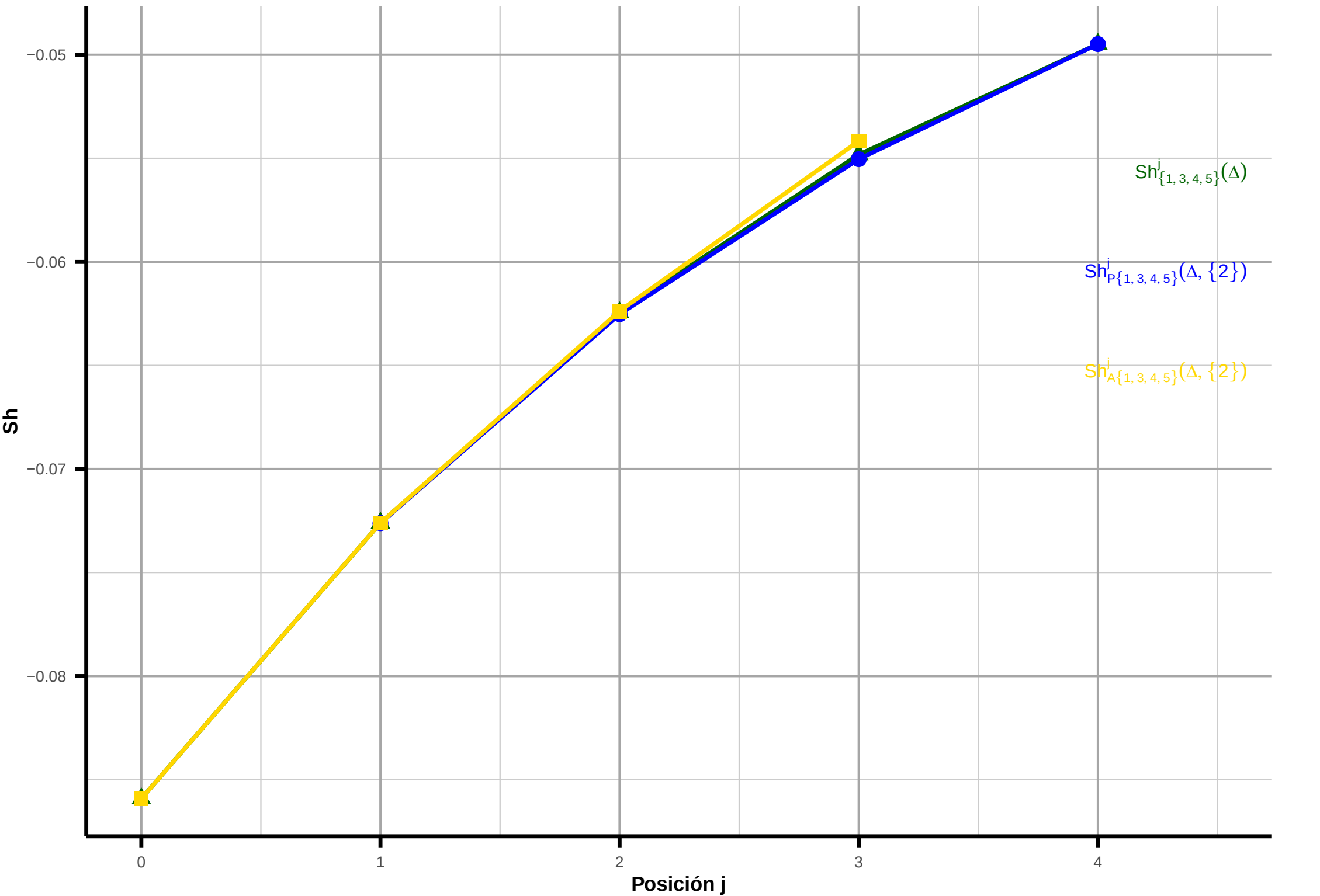
Influencia de Cho [2] sobre Age + Rac + Ris + Sex [1,3,4,5] (instancia fila = 1)
