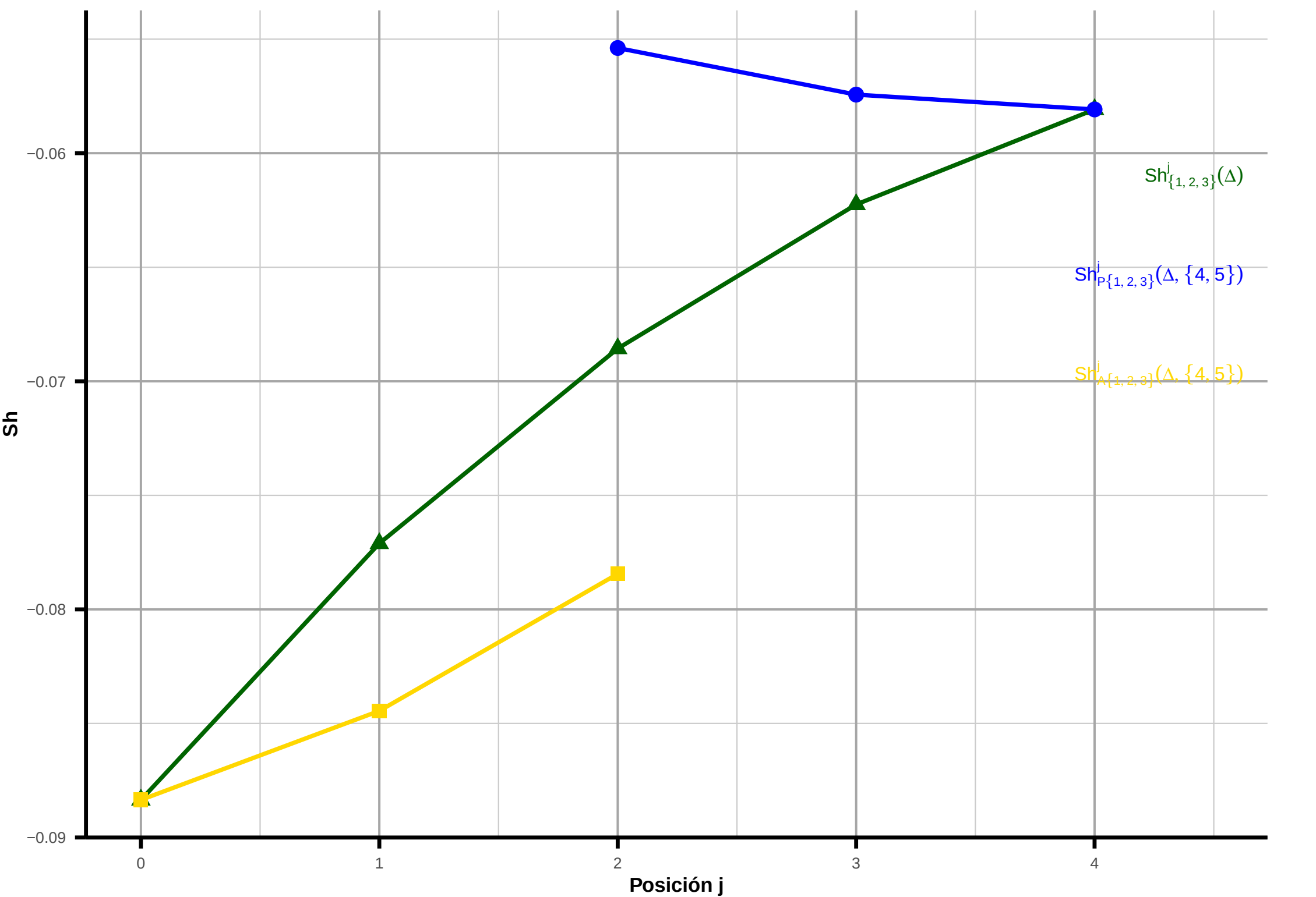
Influencia de Ris + Sex [4,5] sobre Age + Cho + Rac [1,2,3] (instancia fila = 1)
