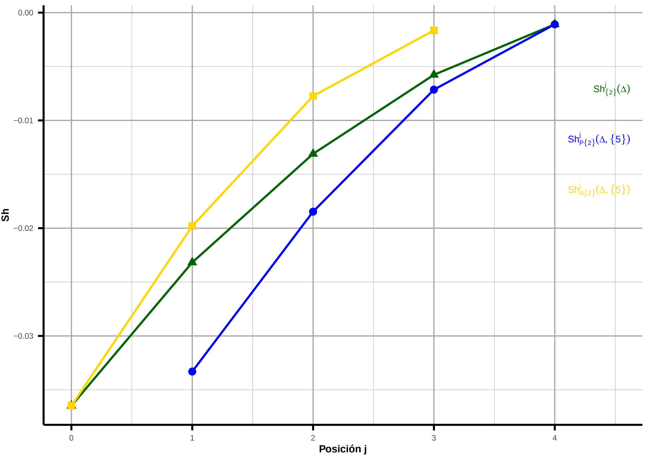
Influencia de Sex [5] sobre Cho [2] (instancia fila = 1)
