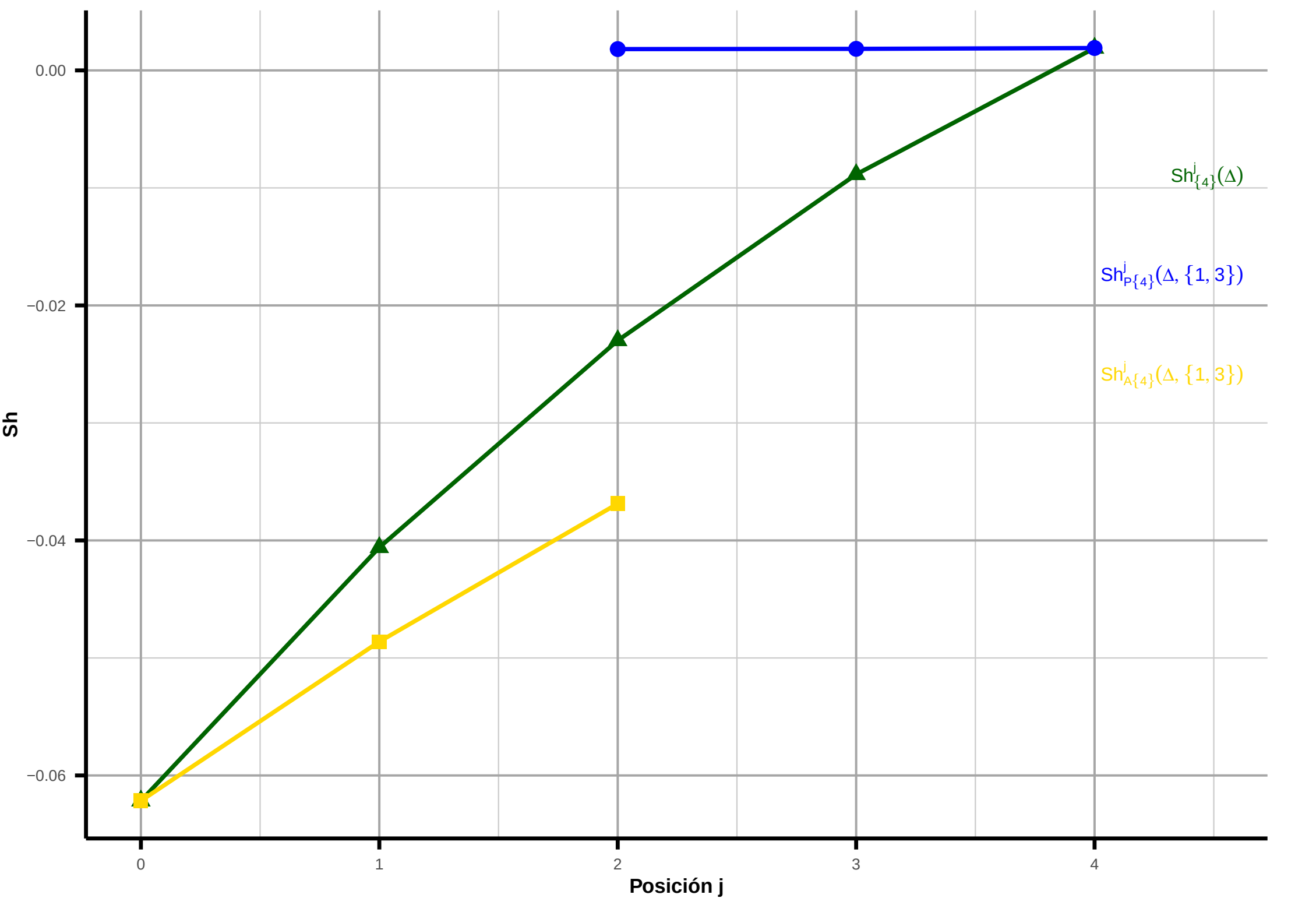
Influencia de Age + Rac [1,3] sobre Ris [4] (instancia fila = 1)
