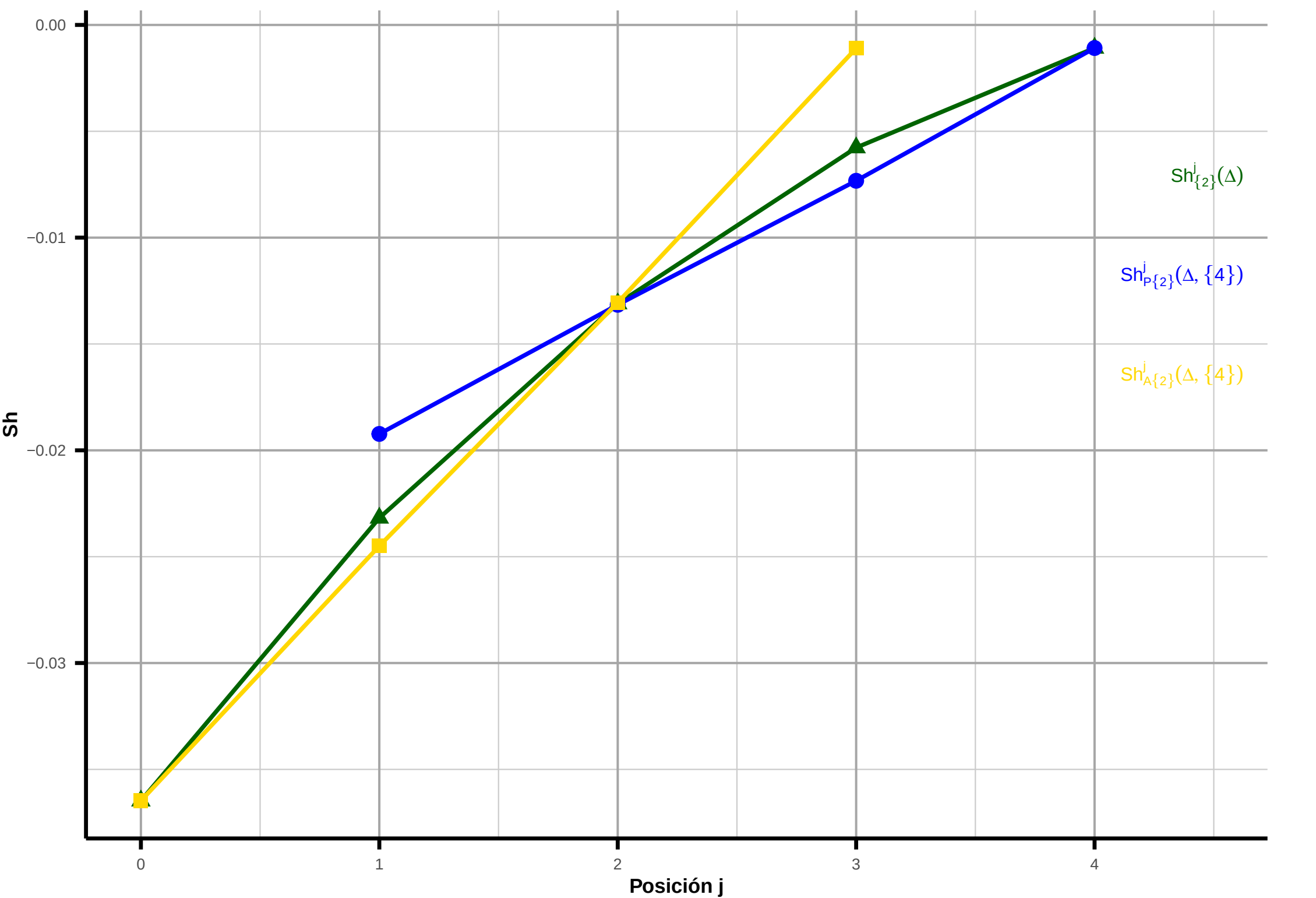
Influencia de Ris [4] sobre Cho [2] (instancia fila = 1)
