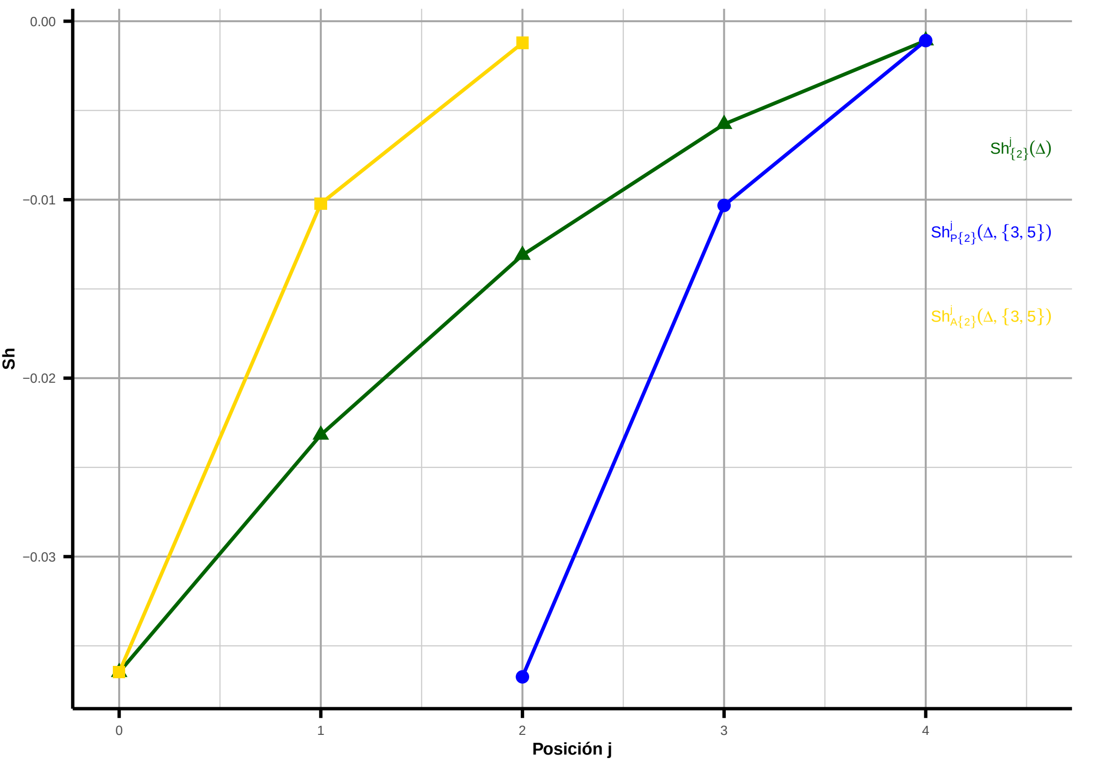
Influencia de Rac + Sex [3,5] sobre Cho [2] (instancia fila = 1)
