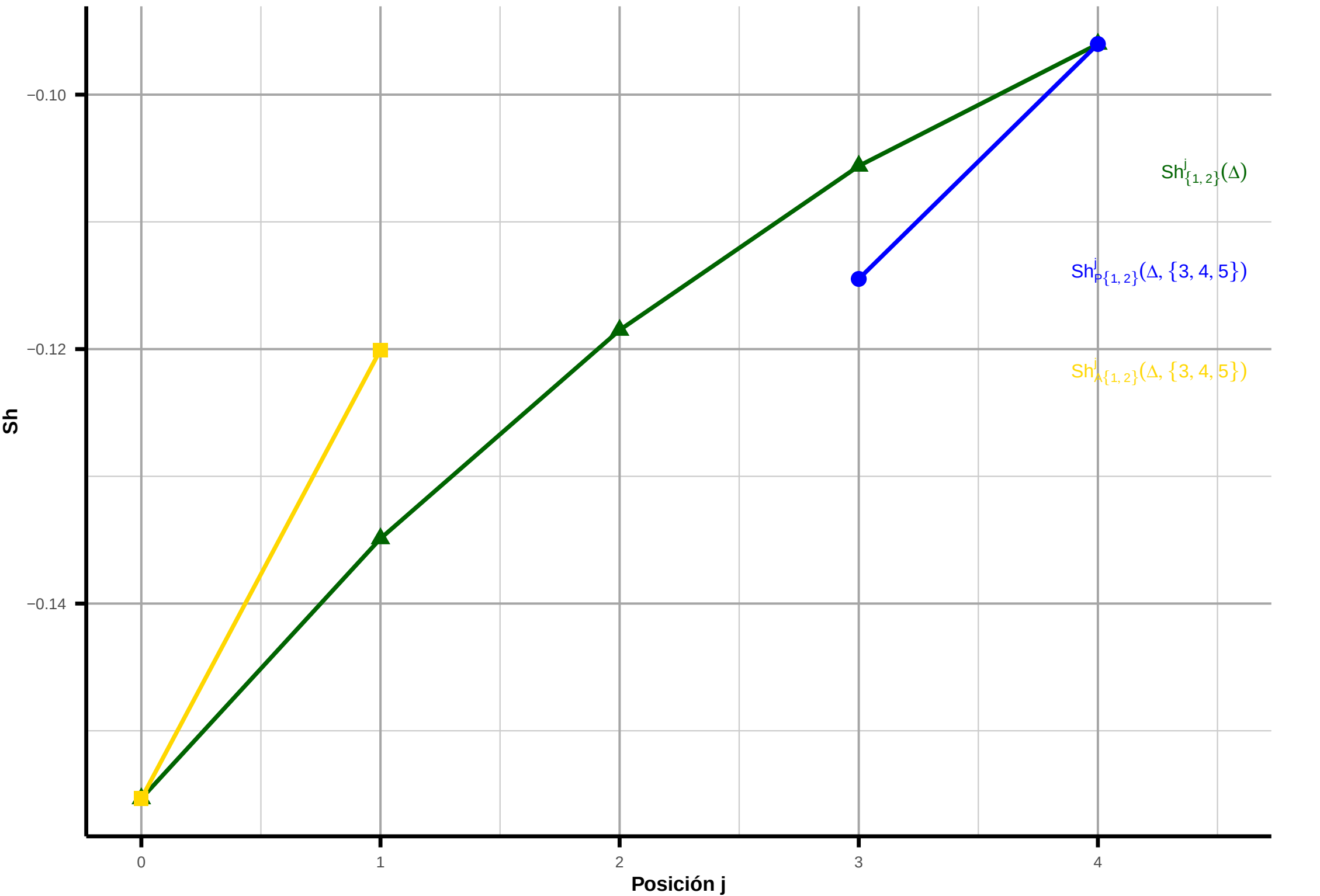
Influencia de Rac + Ris + Sex [3,4,5] sobre Age + Cho [1,2] (instancia fila = 1)
